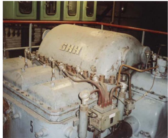
Hochdruckkompressor des Werkes Celanese AG Ehemals Ruhrchemie
